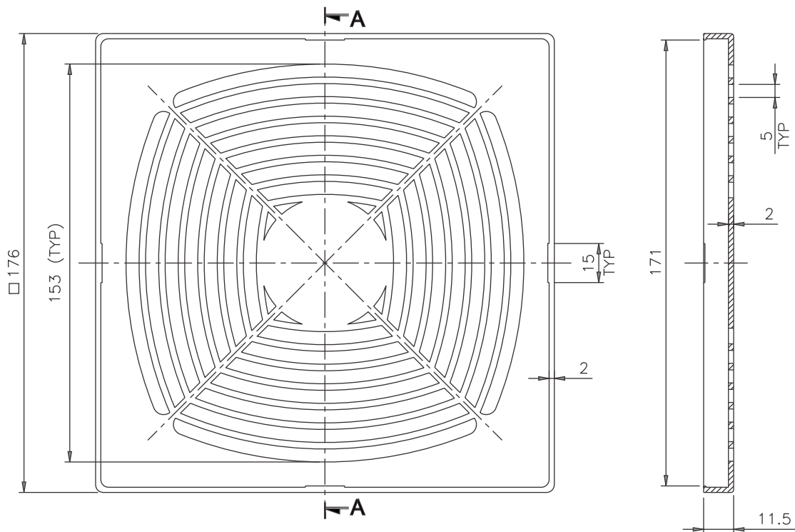
SECTION : A-A
